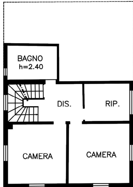
PIANO PRIMO H=2.83
